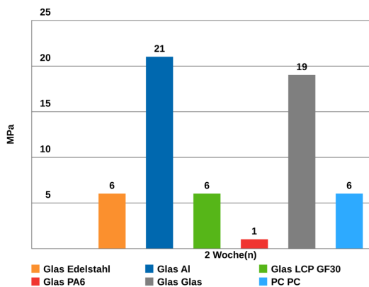
Druckscherfestigkeit nach +85 °C / 85 % r. F. Lagerung, basierend auf DELO-Norm 5
